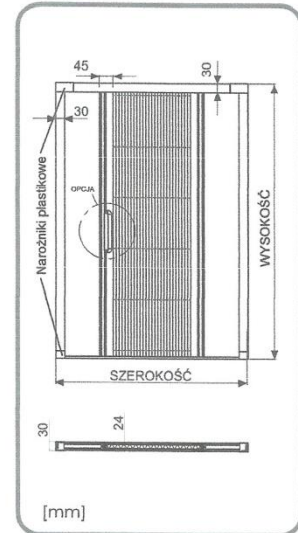
Wymiary profili
